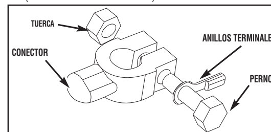
Figura 3. Diagrama de la conexión con anillos terminales
